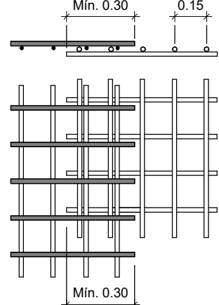
DETALLE TRASLAPO MALLAS Escala 1 : 25
