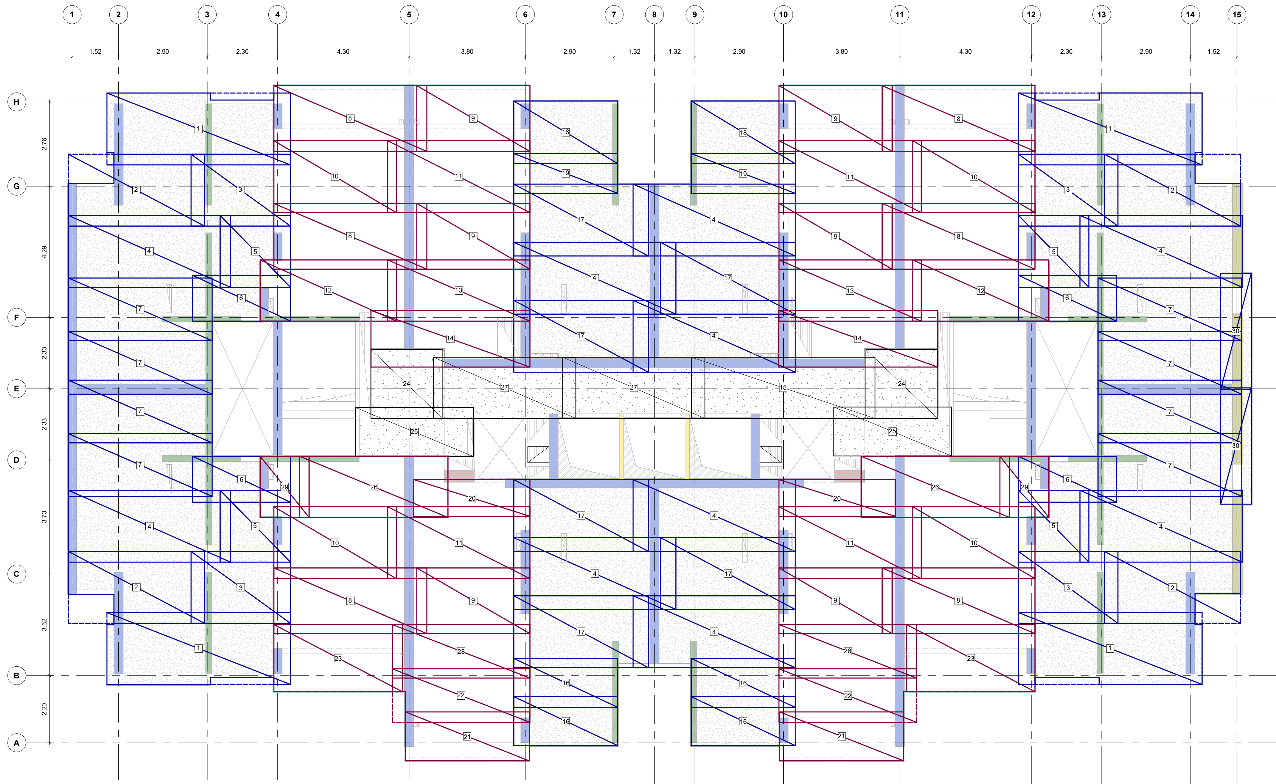
PLANTA DE REFUERZO INFERIOR PISO TIPO 3 ( PISO 23 A PISO 28 ) Escala 1 : 75
