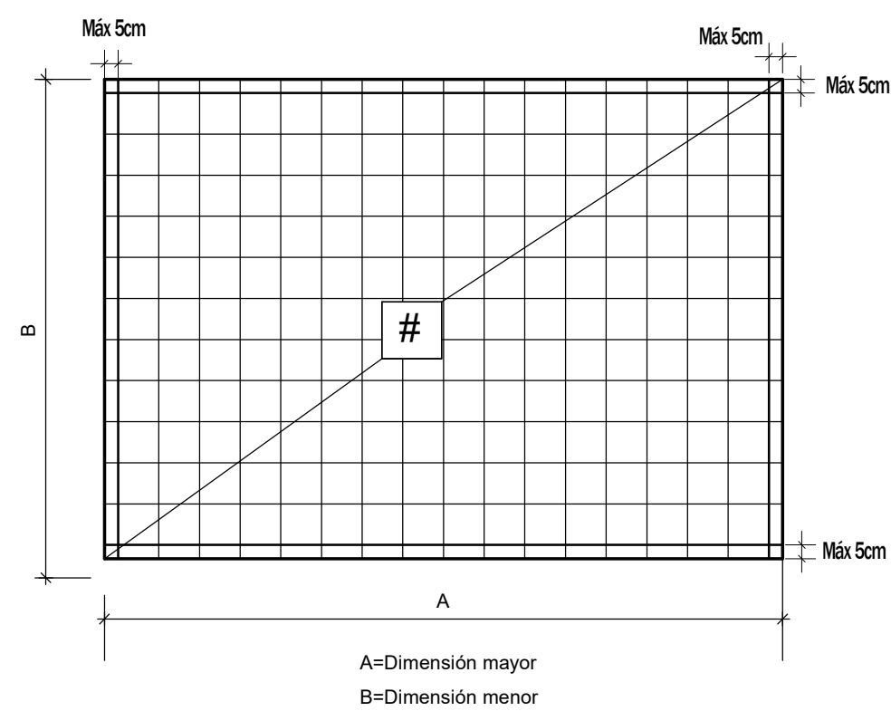
DETALLE CONVENCION MALLAS Escala 1 : 25
